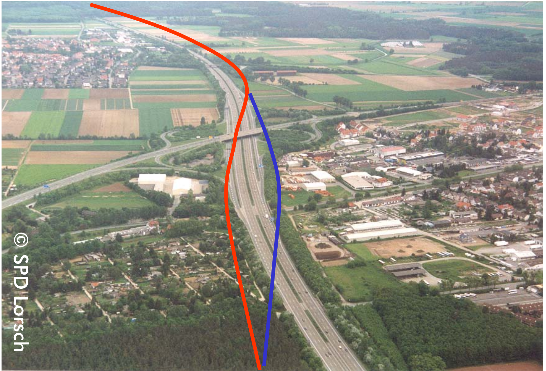
Rot: Entwurfsplanung Blau: ROV-Planung
